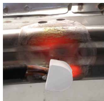
Oldaltag fűtés (ha nem HSS)
